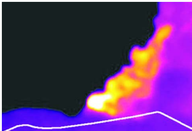
Imagen del volcán Puracé tomada recientemente con cámara geotérmica por el Servicio Geológico Colombiano.
